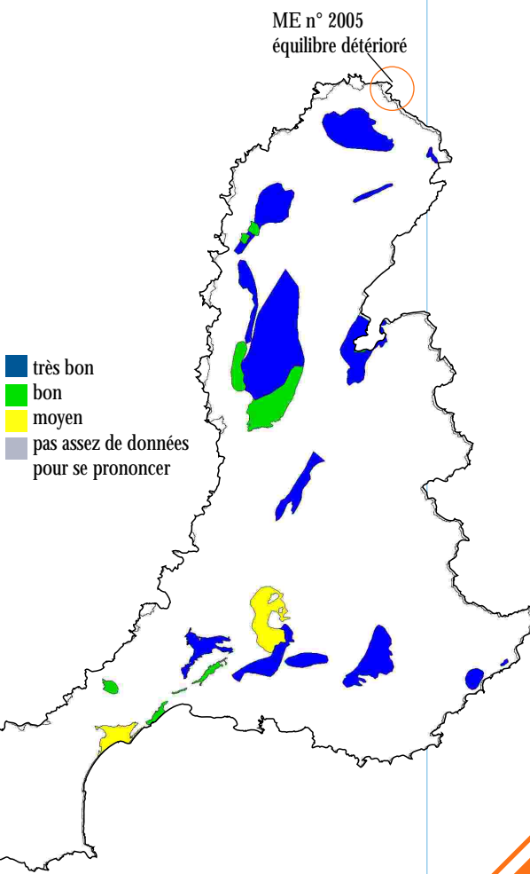
Equilibre de la ressource masses d'eau souterraines sous couverture
