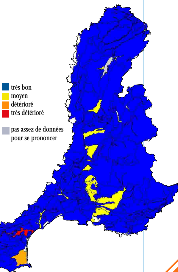
Equilibre de la ressource masses d'eau souterraines à l'affleurement
