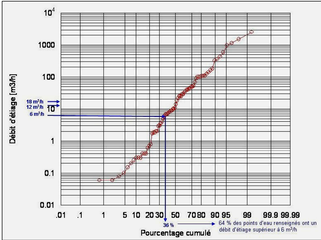
Figure 29 : Distribution statistique des débits d'étéage des sources karstiques non captées ou abandonnées – Courbe des débits classés
