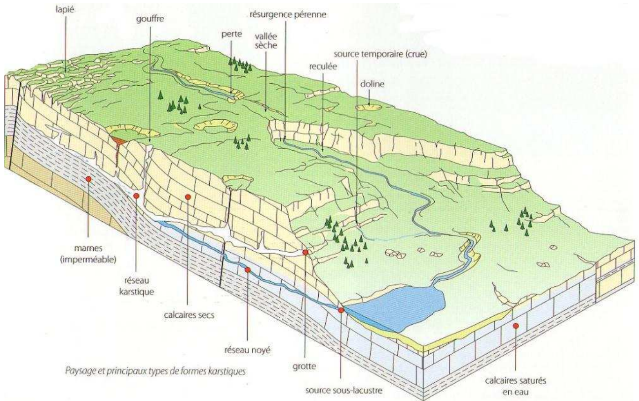
Figure 6 : Paysage et principaux types de morphologies karstiques.
