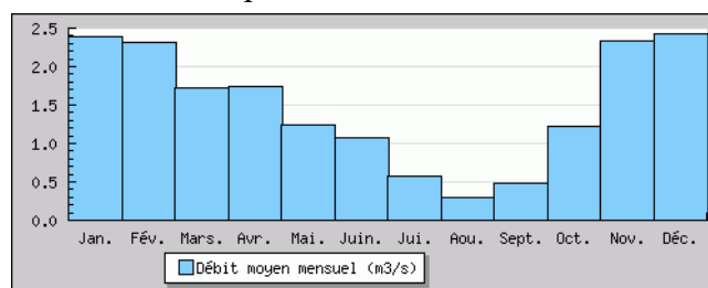
Illustration III.7: Hydrogramme de la Turdine à la station de l' Arbresle [Gobelette] / Banque Hydro
