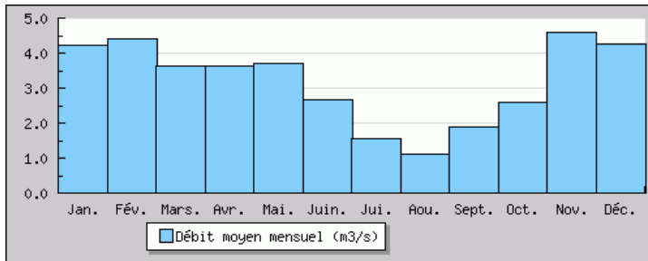
Illustration III.15: Hydrogramme du Gier à la station de Givors / Banque Hydro
