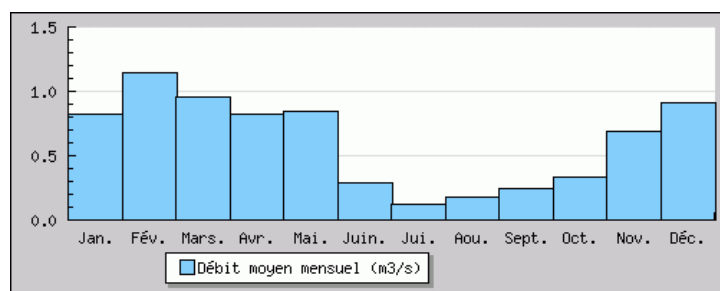
Illustration III.10: Hydrogramme du Garon à la station de Brignais / Banque Hydro
