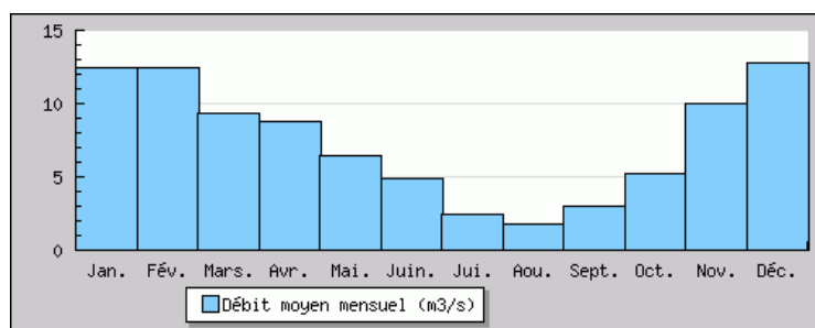
Illustration III.6: Hydrogramme de l'Azergues à la station de Lozanne / Banque Hydro
