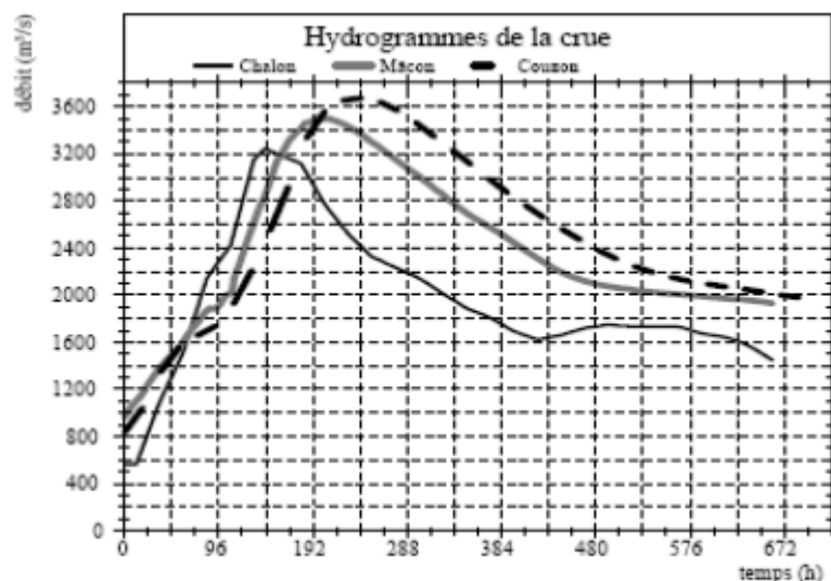
Illustration III.4: Hydrogramme de la crue de référence / Note de Présentation PPRi Saône Moyen
