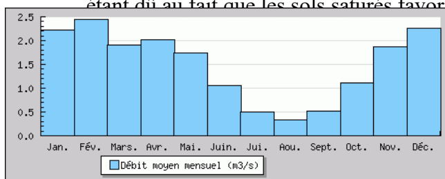
Illustration III.8: Hydrogramme de la Brévenne à la station de Sain-Bel / Banque Hydro
