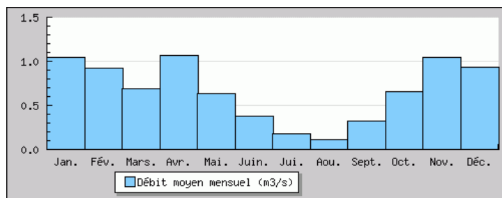
Illustration III.12: Hydrogramme de l'Yzeron à la station de Francheville [Taffignon] / Banque Hydro
