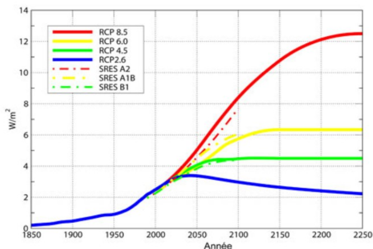
Illustration 28 : Évolution du bilan radiatif de la Terre en W/m^2 selon les différents scénarios du GIEC
