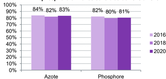
Evolution du rendement d'abattement de l'azote et du phosphore en zones sensibles de 2016 à 2020
