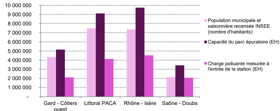
Population, capacité du parc épuratoire et charge entrante mesurée sur les stations de traitement des eaux usées par CTB en 2020 (en nombre d'habitants ou EH)
