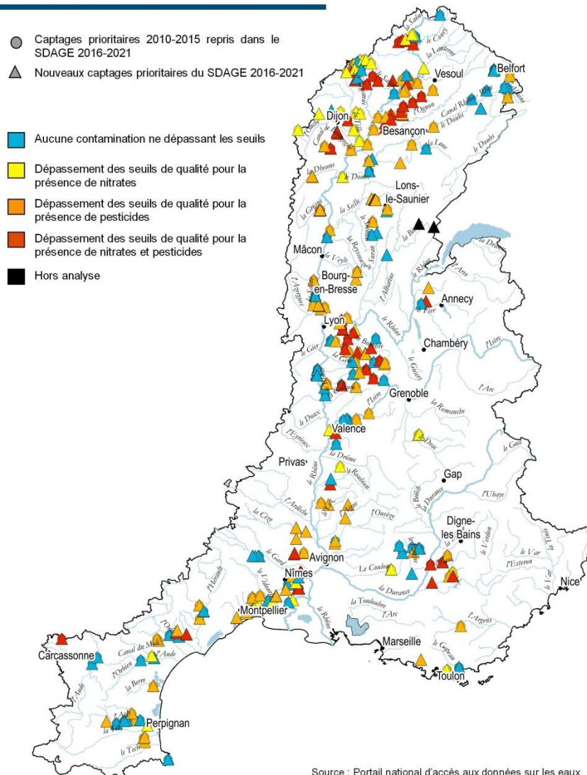
Etat de la contamination par les nitrates et/ou pesticides sur les 269 captages prioritaires du SDAGE 2016-2021 (données 2015-2020)
