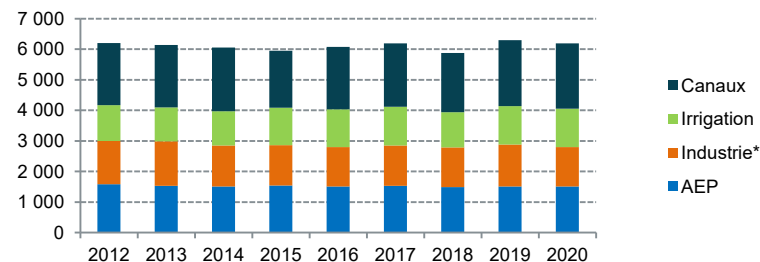
Évolution des volumes prélevés en eaux superficielles et souterraines par usage (en millions de m 3 ) - hors CNPE en circuit ouvert
