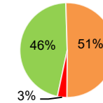
Répartition sur l'ensemble du bassin Rhône-Méditerranée
