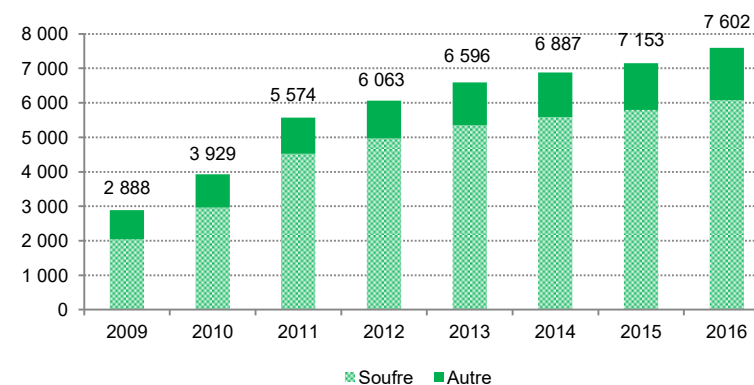
Évolution des ventes de produits autorisés en agriculture biologique (en quantité de substances actives exprimées en tonnes)
