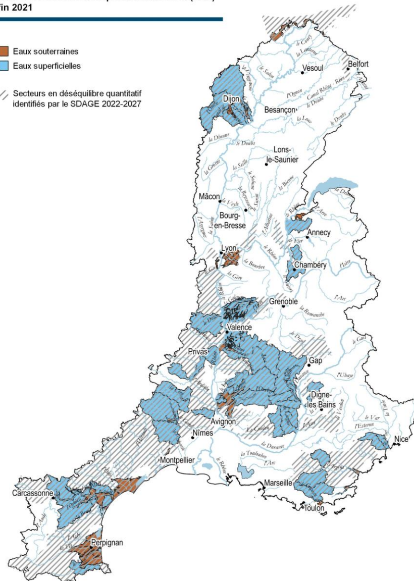
Classement en zone de répartition des eaux (ZRE) à fin 2021
