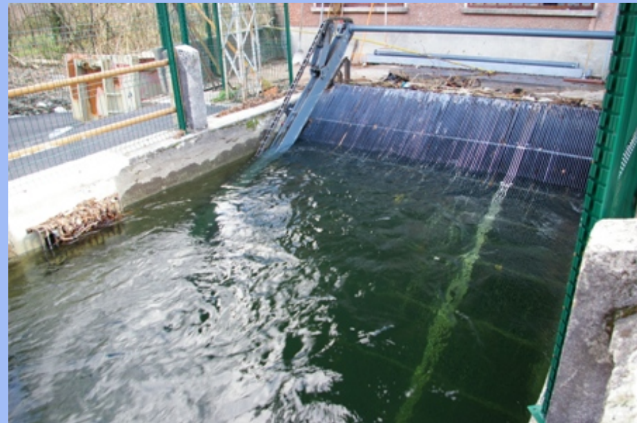
Dévalaison 2010 grille 2 cm Exutoire latéral
