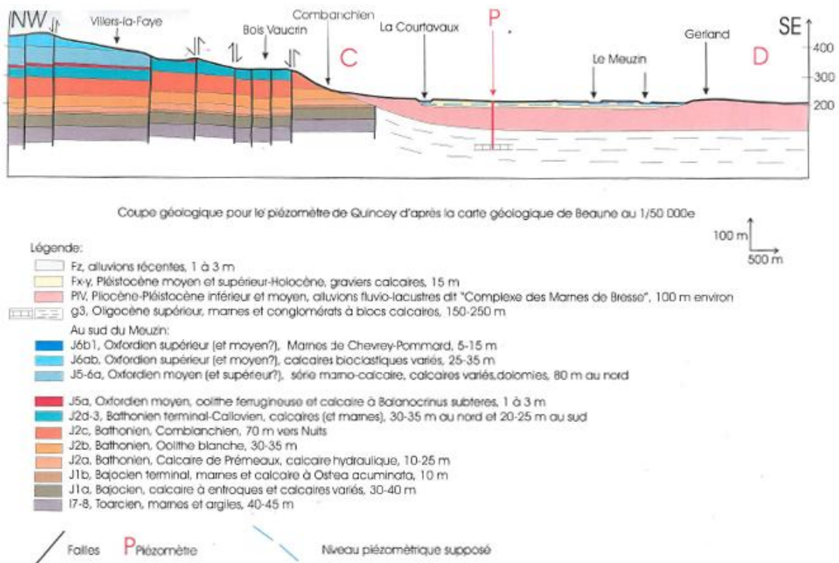
Figure 94 : Coupe passant par la source de Courtavaux (DREAL Bourgogne)
