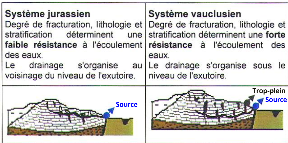
Figure 14 : Systèmes karstiques jurassien et vaclusien (D'après Marsaud 1996)
