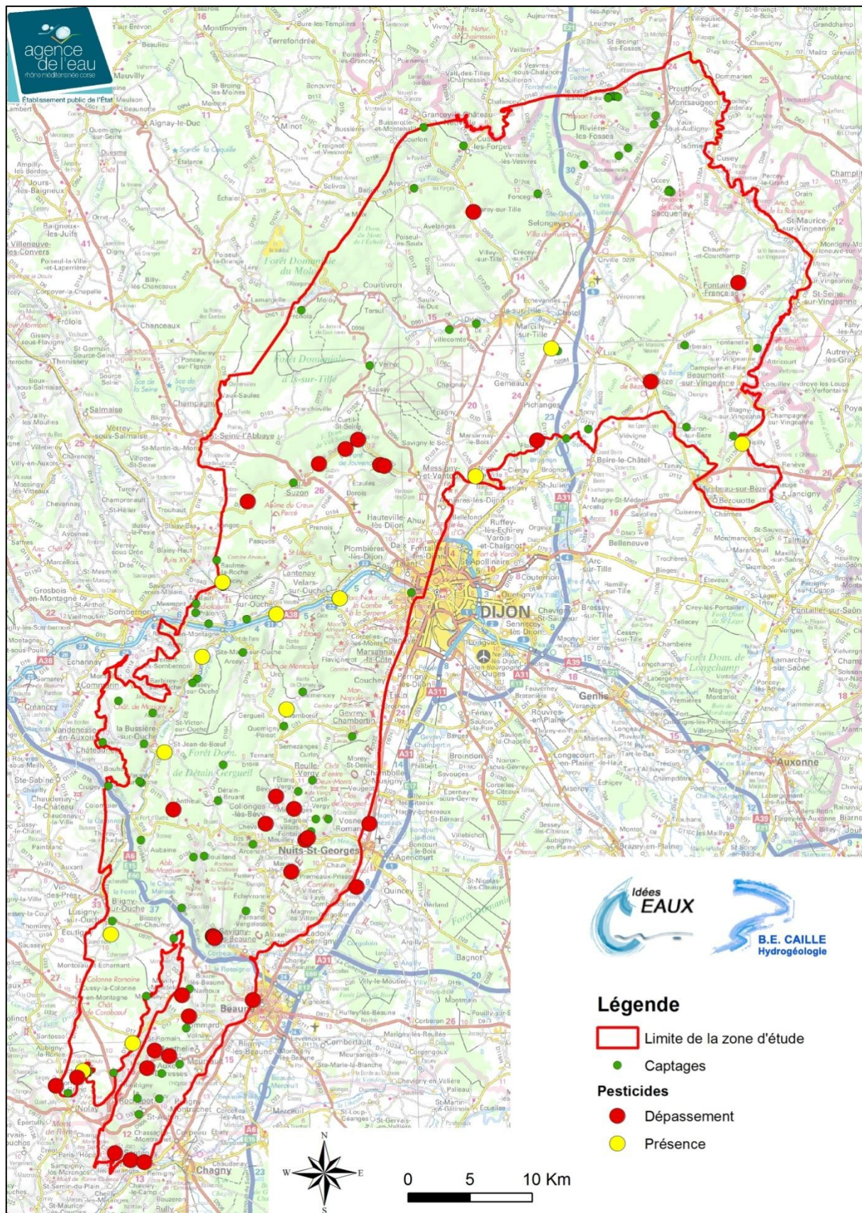
Figure 47 : Répartition des présences et dépassements de pesticides par captage sur les eaux brutes
