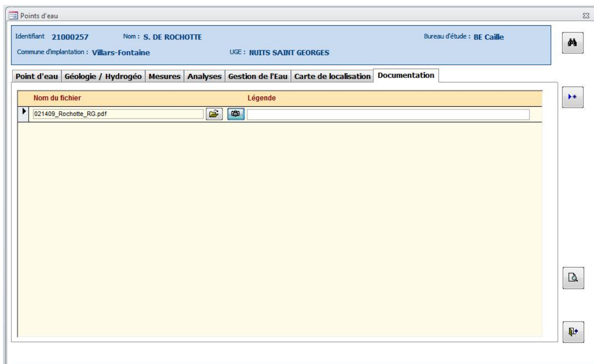
Figure 22 : Onglet « Documentation »
