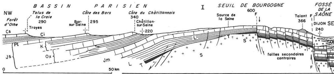
Figure 4 : Coupe géologique du Seuil de Bourgogne (P. Rat)
