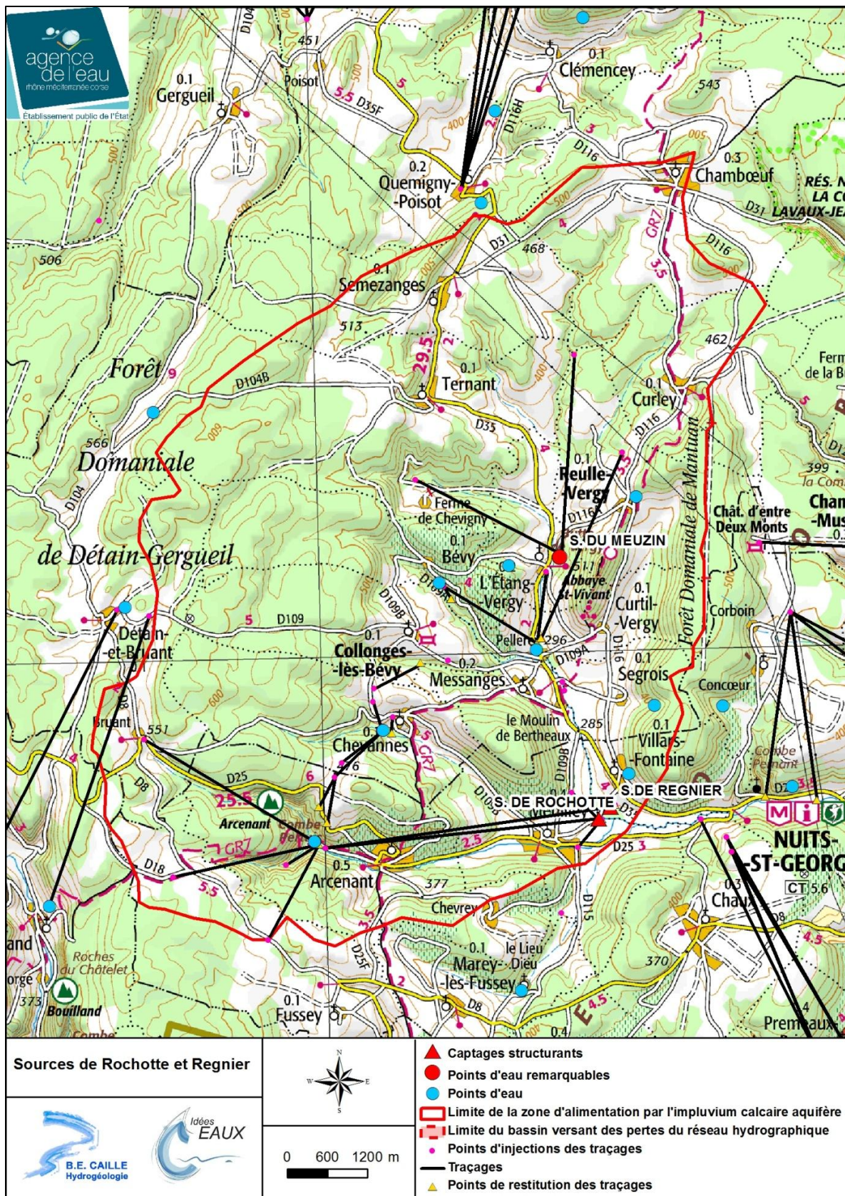
Figure 69 : Limite du bassin d'alimentation des sources Rochotte et Regnier sur fond IGN au 1/100 000 ème
