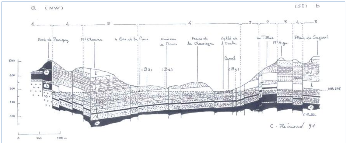
Figure 85 : Coupe géologique transversal recoupant la vallée de l'Ouche
