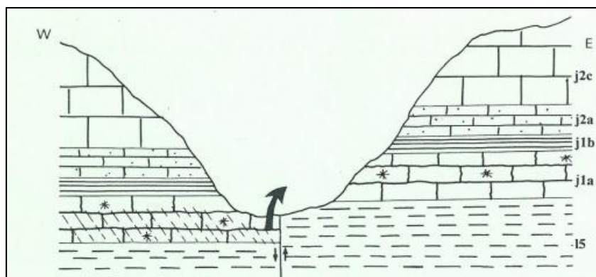
Figure 80 : Coupe géologique au niveau de la source de Sainte-Foy (d'après JP REBOUILLAT en 1984)
