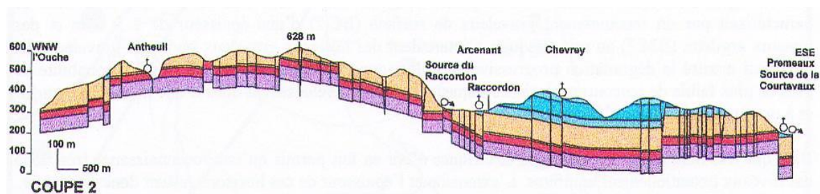
Figure 68 : Coupe géologique du secteur des sources Rochotte et Regnier (D'après la thèse de P. Corbier )
