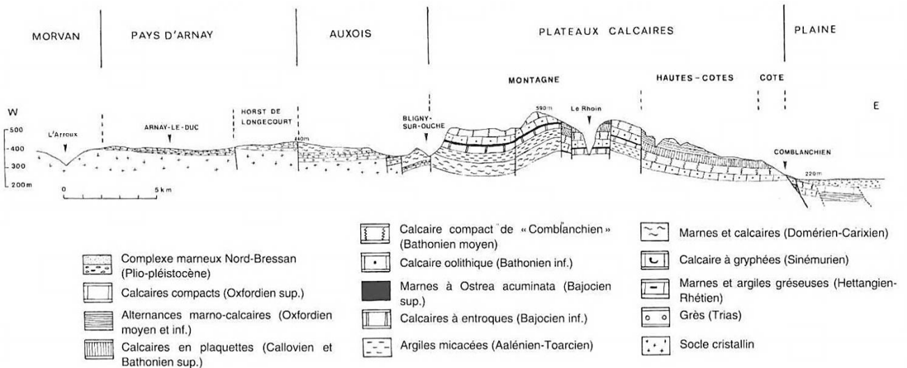
Figure 5 : Coupe de la Côte (INRA)
