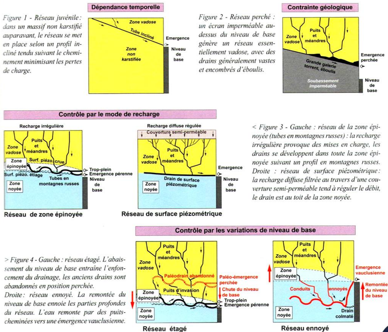
Figure 13 : Modèle de spéléogénèse (D'après Philippe Audra, dans « Grottes et karsts de France », Ed. Karstologia Mémoires, 2010)
